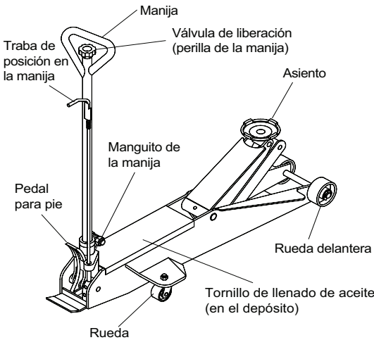
Figura 2: Componentes de los modelos 25057 y 25107
