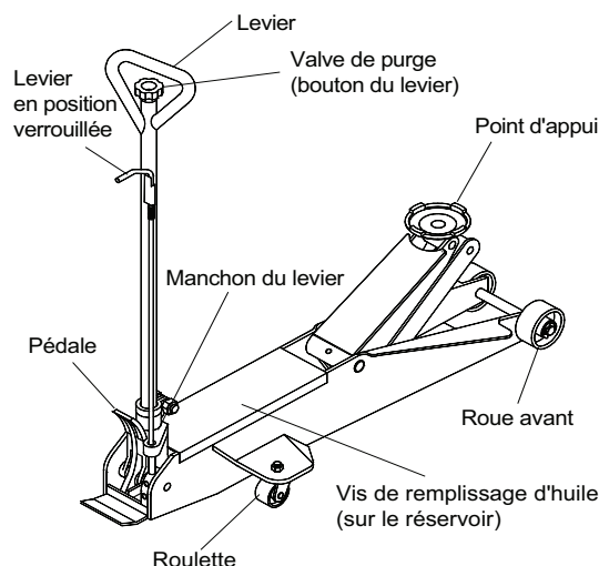
Figure 1: Composants des modèles 25057 et 25107
