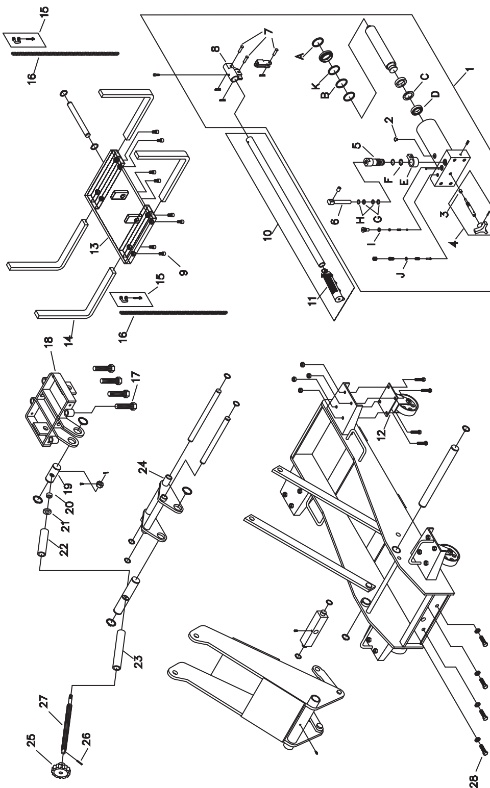
Figura 2: Ilustración de piezas de repuesto para el modelo 43000
