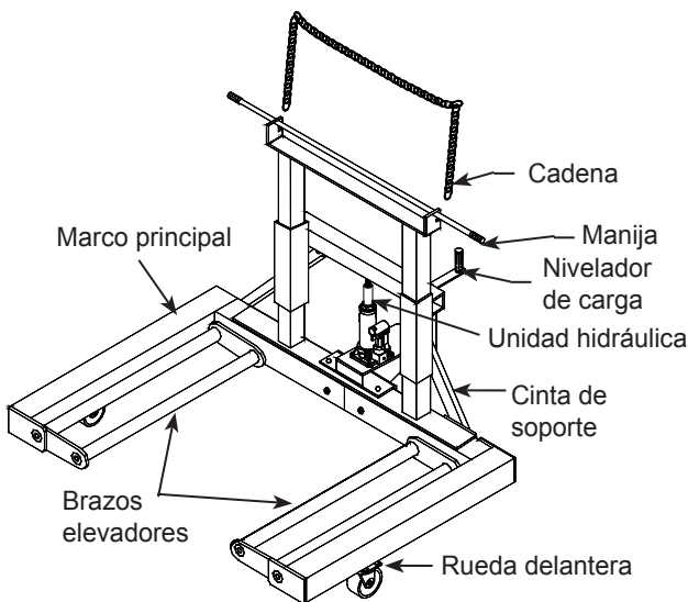
Figura 2: Componentes de la plataforma rodante 47053
